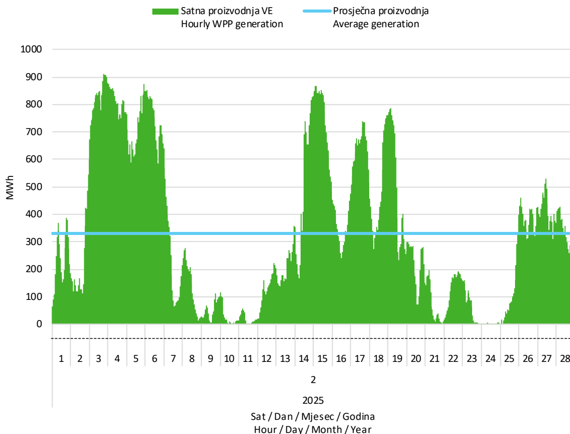
Slika 2 Satna proizvodnja svih vjetroelektrana u veljači 2025. godine
