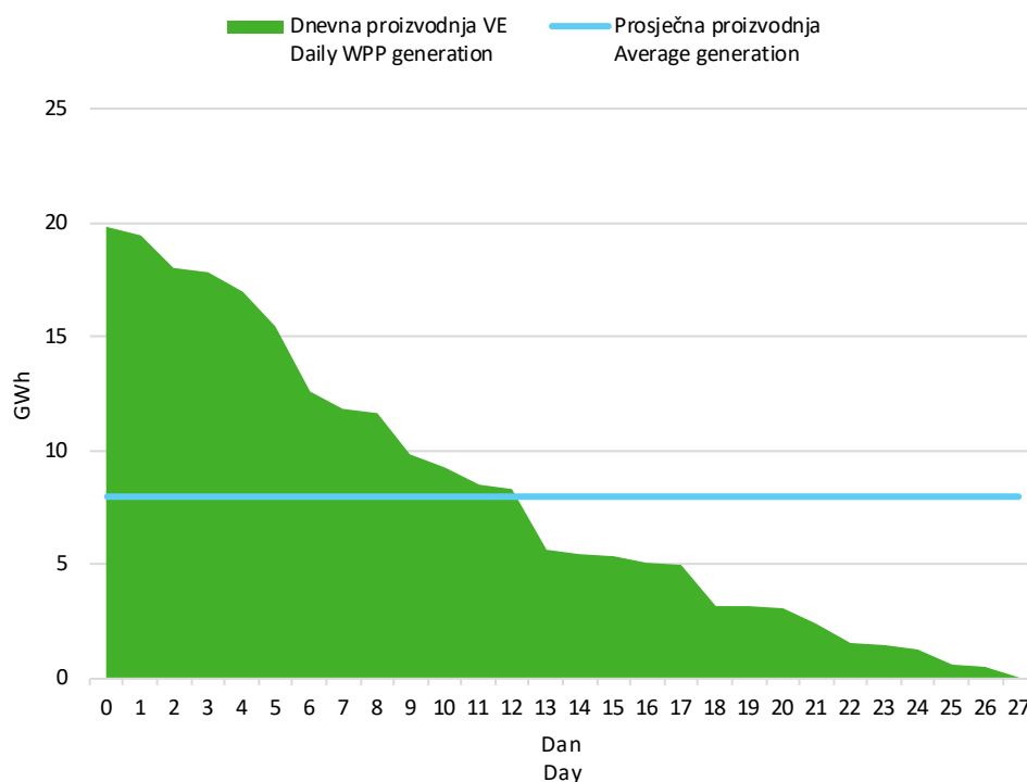
Slika 6 Krivulja trajanja dnevne proizvodnje vjetroelektrana u veljači 2025. godine
