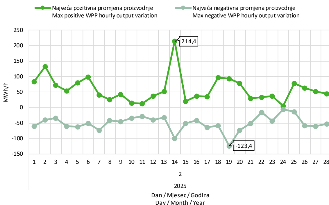
Slika 9 Maksimalna pozitivna i maksimalna negativna promjena satne proizvodnje VE u veljači 2025. godine
