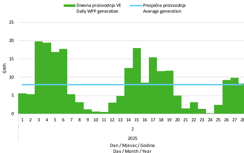
Slika 5 Dnevna proizvodnja svih vjetroelektrana u veljači 2025. godine
