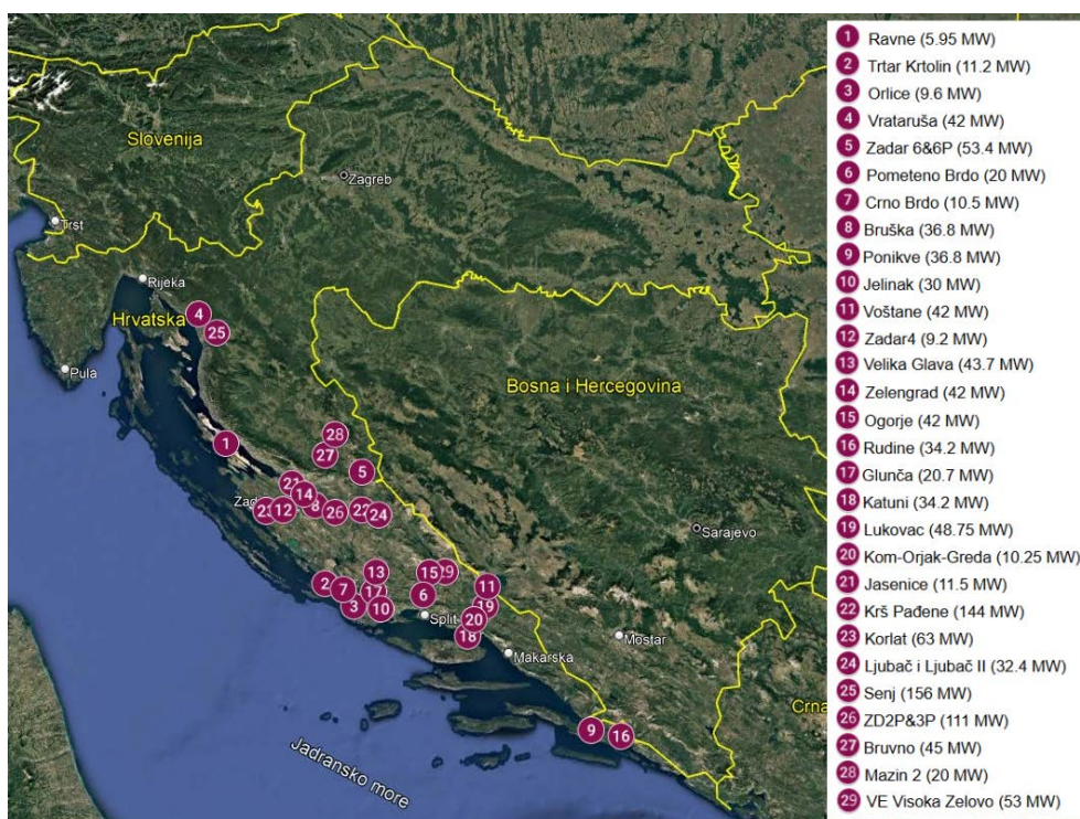
Slika 1 Lokacije VE u Hrvatskoj
