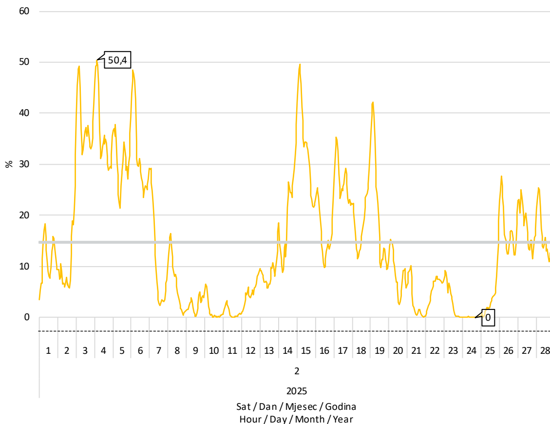
Slika 8 Udio proizvodnje vjetroelektrana u pokrivanju satnog opterećenja elektroenergetskog sustava u veljači 2025. godine
