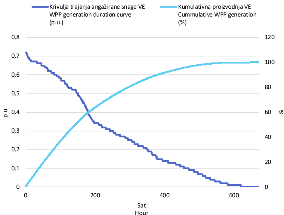
Slika 3 Krivulja trajanja angažirane snage svih VE i kumulativna proizvodnja VE u veljači 2025. godine u jediničnim vrijednostima
