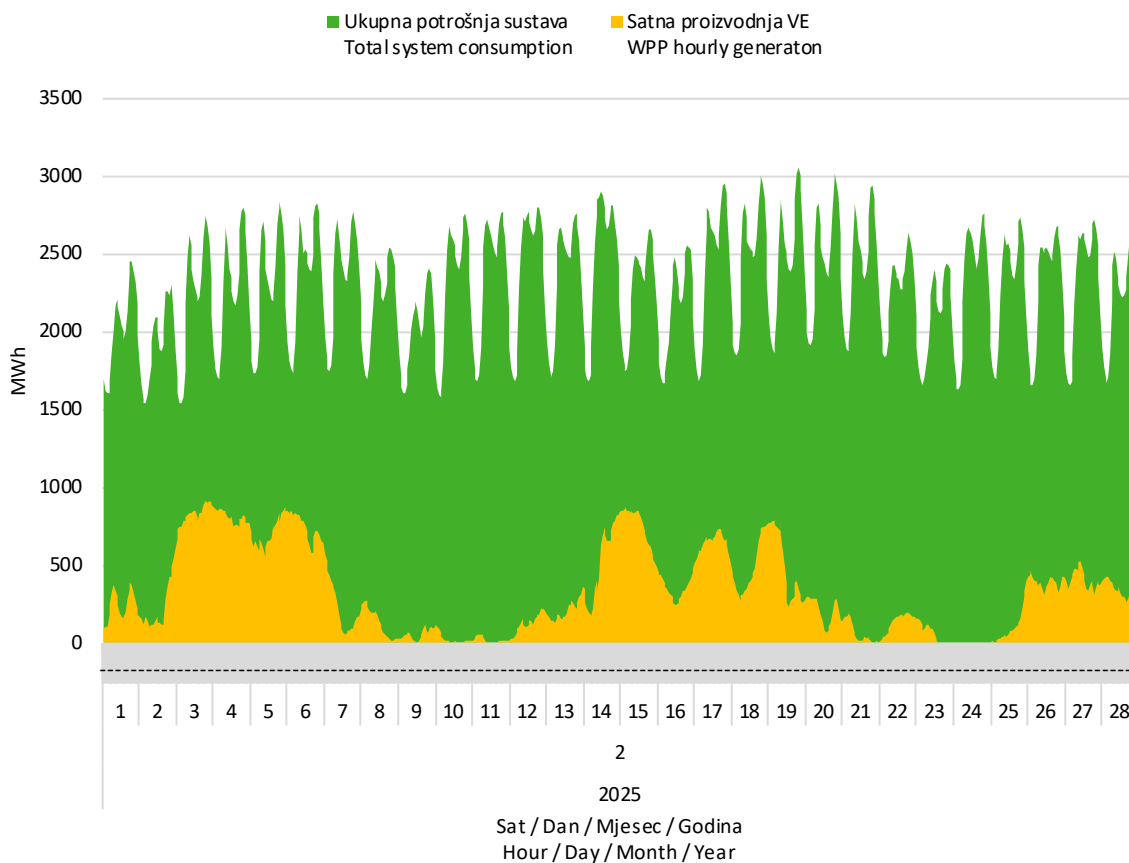
Slika 7 Usporedba satnog dijagrama opterećenja sustava i proizvodnje vjetroelektrana u veljači 2025. godine
