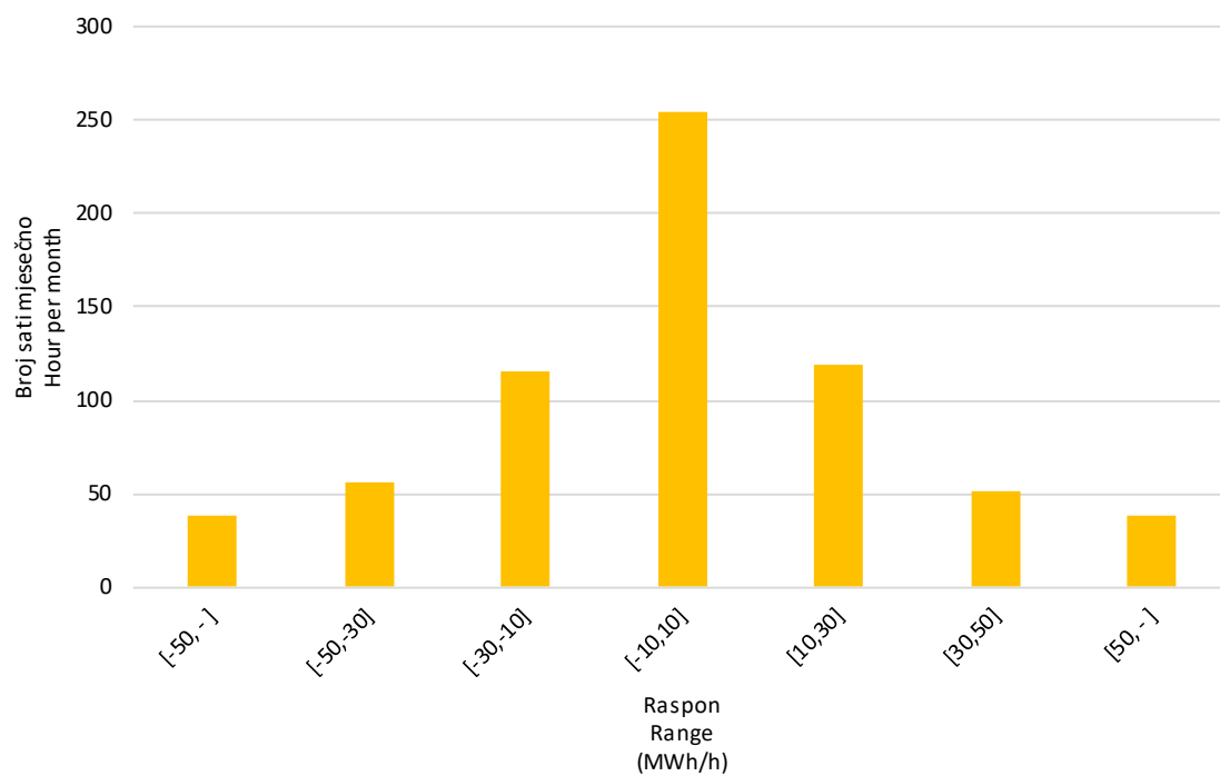
Slika 10 Statistička raspodjela satnih promjena proizvodnje VE u veljači 2025. godine
